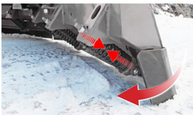
Snijkant met tripveren
